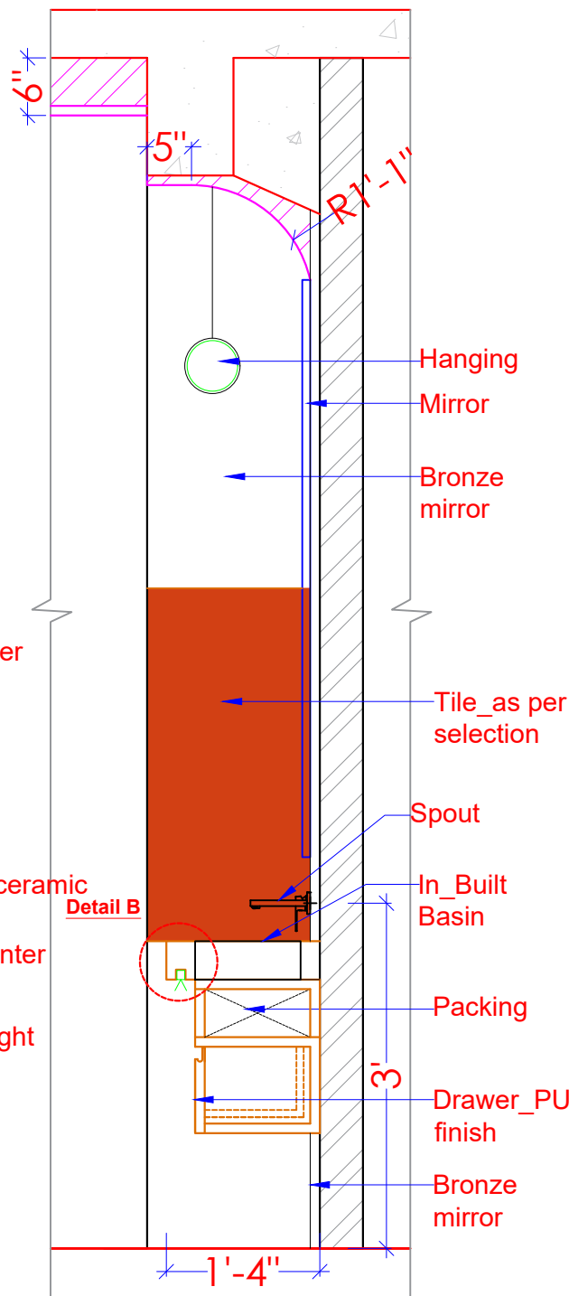
ELEVATION - b
